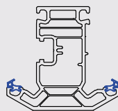
103365 76mm Casement Sash/T Mullion
